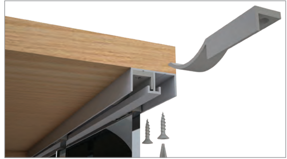
Stoplama Plastiği Stopper
