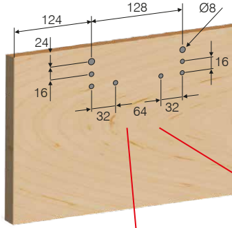
DİŞ KAPAK EXTERNAL DOOR
