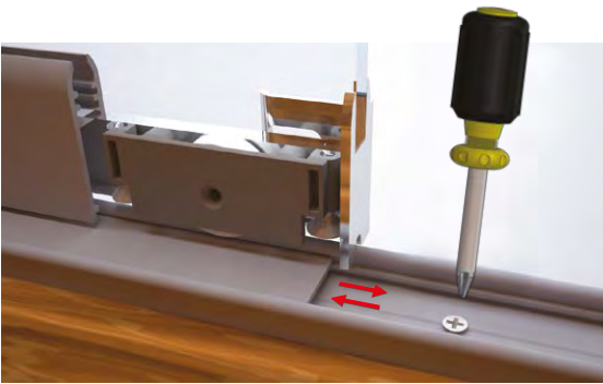
Alt ray ve kapama profili (Kapama profili montaj vidalarını gizlemek için kullanılır.) Cover profile for lower rail
