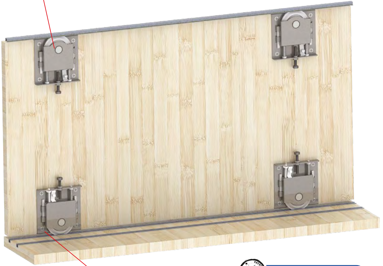
Tutucu mandal Lock pin
