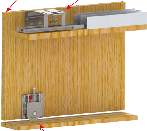
DIŞ KAPAK EXTERNAL DOOR
