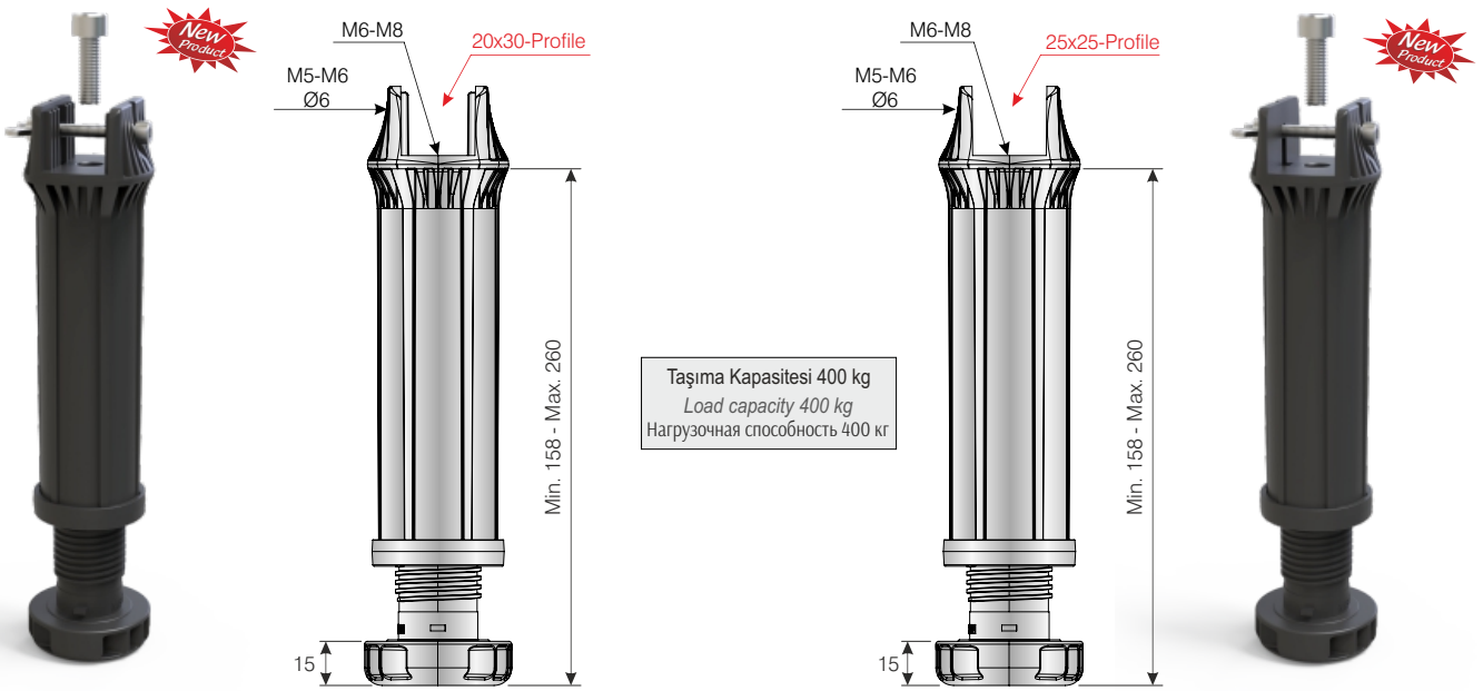
104-01-47 104-01-48 M6 M8 20 x 30 mm Profil 20 x 30 mm Profile 20 x 30 mm профиль
