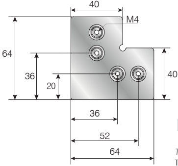
110-22-01 Kalınlık 3mm Thickness 3mm Толщина 3 мм
