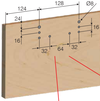
DIŞ KAPAK EXTERNAL DOOR НАРУЖНАЯ ДВЕРЬ
