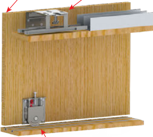
DIŞ KAPAK EXTERNAL DOOR НАРУЖНАЯ ДВЕРЬ
