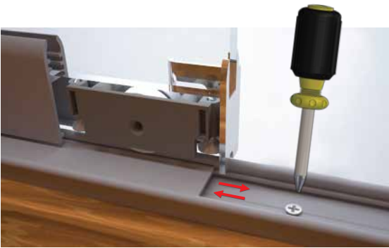
Alt ray ve kapama profili (Kapama profili montaj vidalarını gizlemek için kullanılır.) Cover profile for lower rail Крышка нижней направляющей
